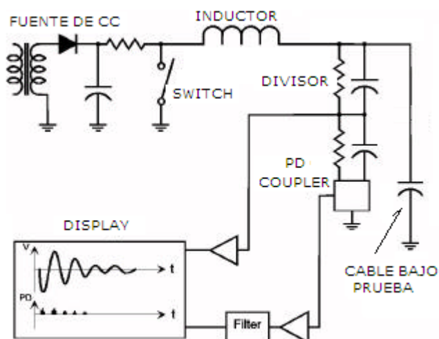
Esquema eléctrico del sistema DAC de Ondas Oscilantes Amortiguadas
